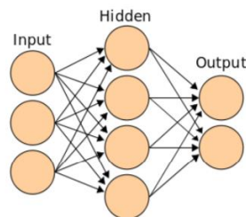
Gambar 3. Pemodelan JST[6]
