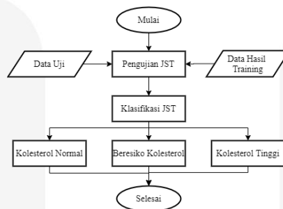
Gambar 8. Klasifikasi JST
