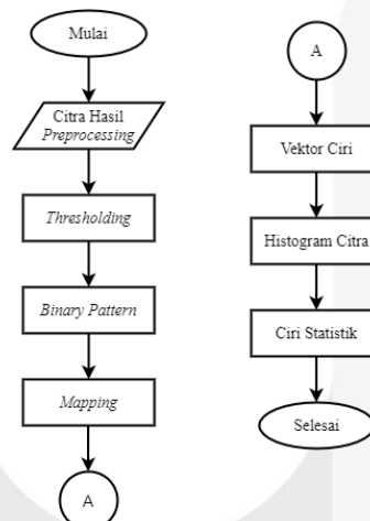
Gambar 6. Ekstraksi Ciri
