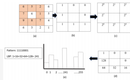
Gambar 2. Operasi LBP[9]
