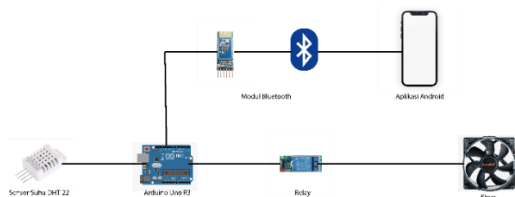
Gambar 1 Sistem Arsitektur
