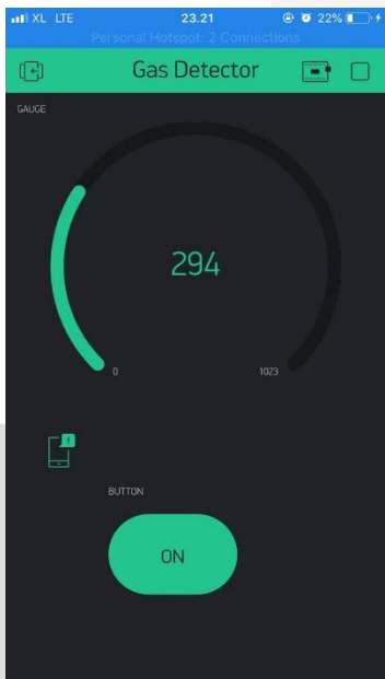
Gambar 4.8 Tampilan Antarmuka
