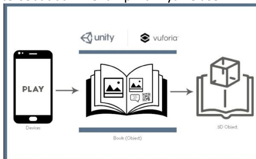
Gambar 3.1 Sistem Arsitektur
