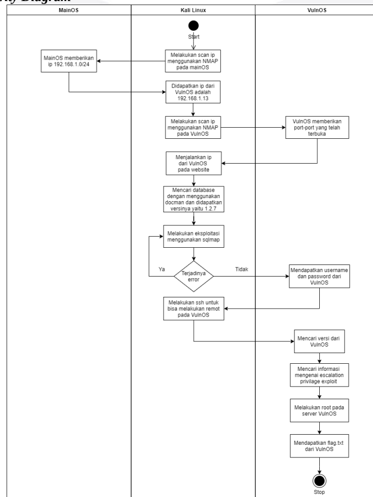
Gambar 4 Activity Diagram pada Walkthrough
