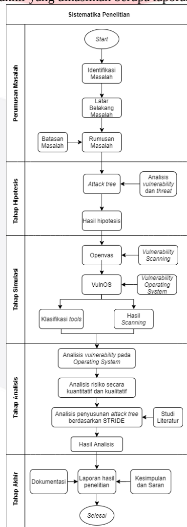
Gambar 2 Sistematika Penelitian
