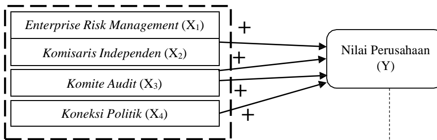
Gambar 2.1 Kerangka Pemikiran
