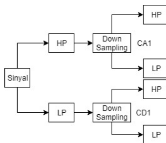
Gambar 4. Dekomposisi Sinyal
