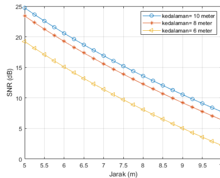
Gambar 4. 3 Hasil Simulasi SNR terhadap Jarak
