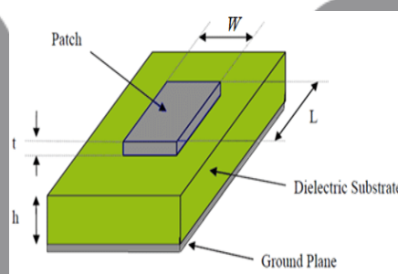
Gambar 2.1 Antena Mikrostrip Persegi [11].
