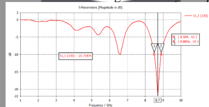
Gambar 4.4 Nilai Return Loss Antena Patch Persegi Proximity Coupled Untuk 4 Section Setelah Optimasi.
