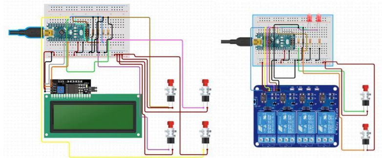
Gambar 3.2 Perancangan Rangkaian
