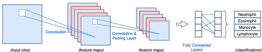
Gambar 6. Arsitektur CNN
