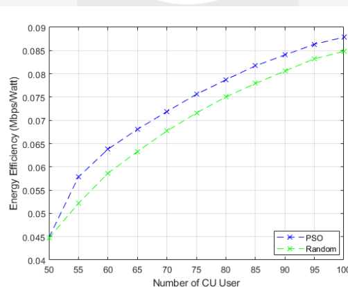
Gambar 4. Grafik Efisiensi Energi
