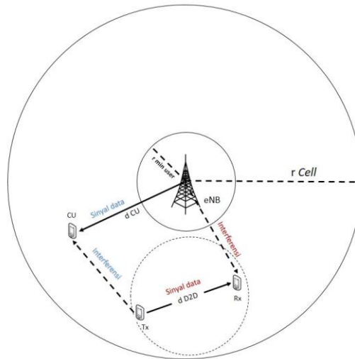
Gambar 1. Pemodelan Sistem.
