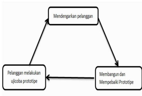
Gambar 1. Metode Prototipe
