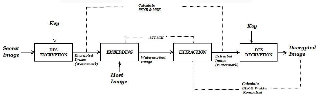
Gambar 1. Diagram Alir Model Perancangan Sistem
