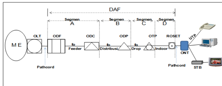
Gambar I.1 Arsitektur FTTH
