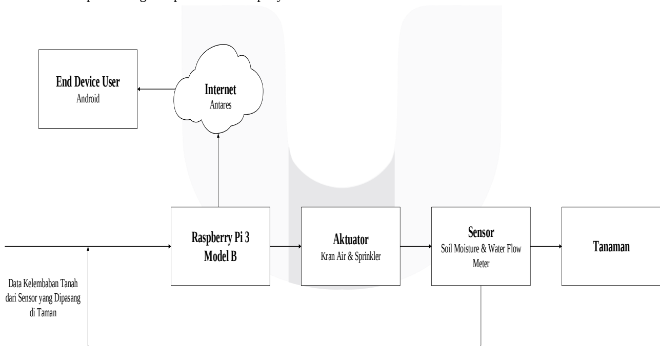
Gambar 3. 2 Blok Diagram Sistem Otomatis
