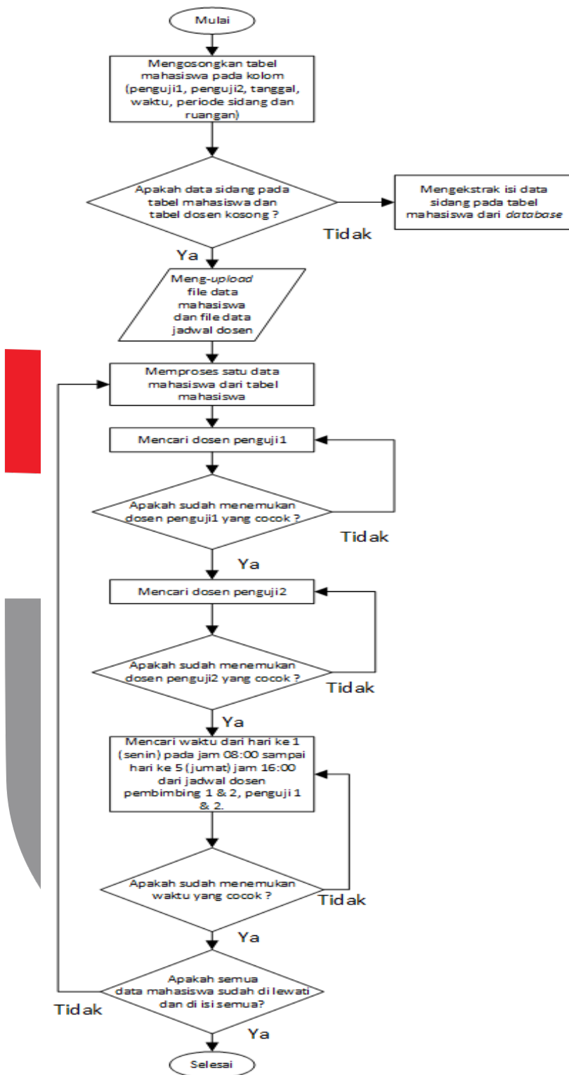
Gambar 3. 14 Flowchart Proses Metode Jadwal Sidang Proyek Akhir
