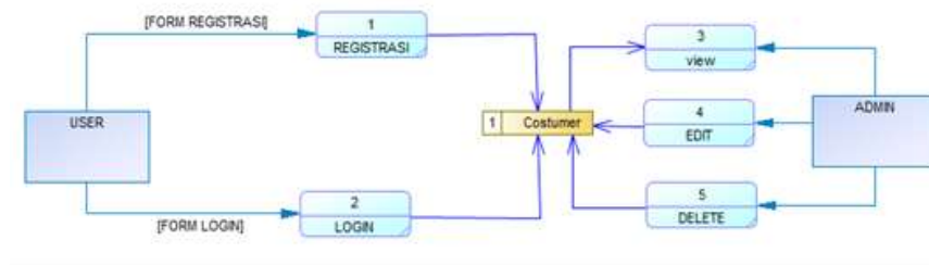
Gambar 3 DFD
