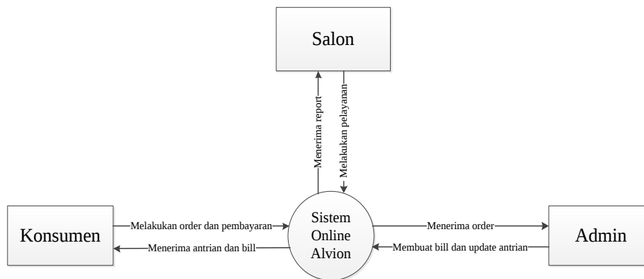
Gambar 1 Konteks Diagram
