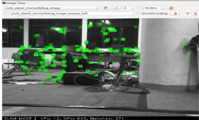
Gambar 5. Tampilan ORB SLAM dalam memproses
