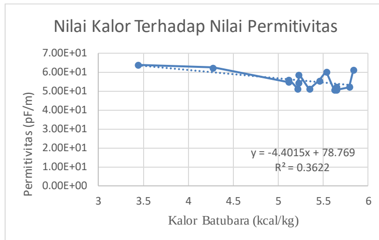
Gambar 5 Grafik Penentuan Nilai Permittivitas
