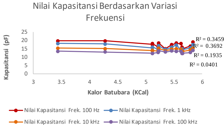
Gambar 3 Grafik nilai kapasitansi berdasarkan variasi frekuensi
