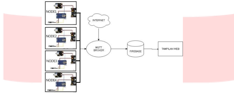
Gambar 3 Desain Sistem
