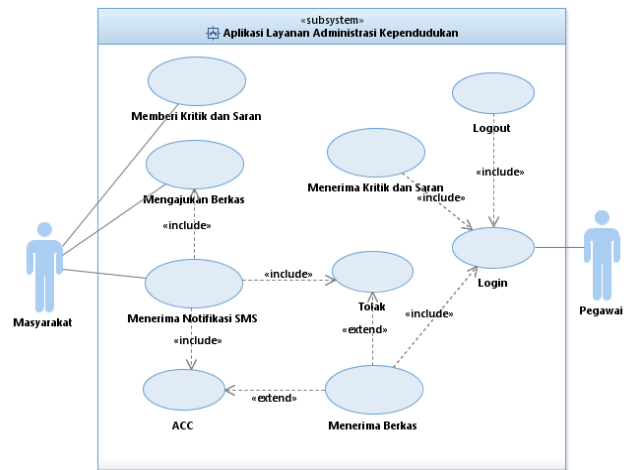
Gambar 1.1 : Use Case Diagram Aplikasi
