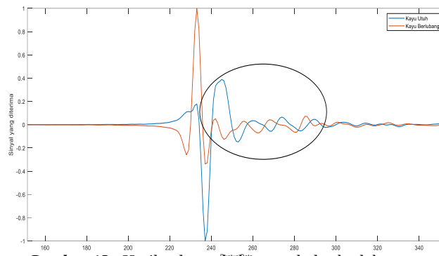
Gambar 13. Hasil pulsa pada kayu utuh dan berlubang.
