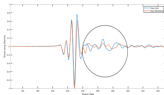
Gambar 8. Hasil pulsa pada kayu utuh dan berlubang.
