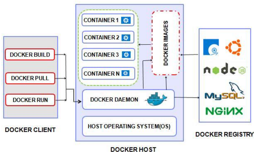
Gambar 2.3.1. Arsitektur Docker [10]
