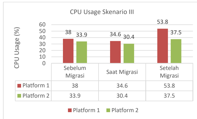
Gambar 5 Grafik CPU Usage Skenario III
