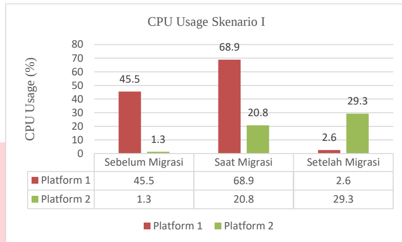
Gambar 3 Grafik CPU Usage Skenario 1
