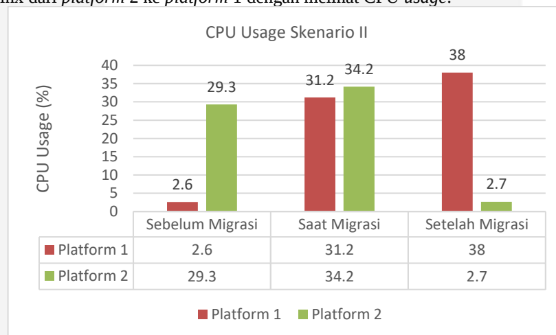
Gambar 4 Grafik CPU Usage Skenario II
