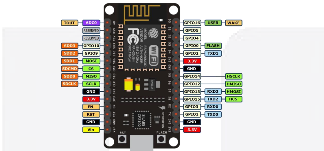
Gambar II-5 . NodeMCU
