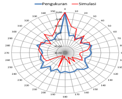
Gambar 15 Pola radiasi elevasi simulasi dan pengukuran
