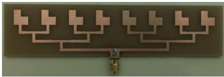
Gambar 7 Realisasi antenna tampak depan
