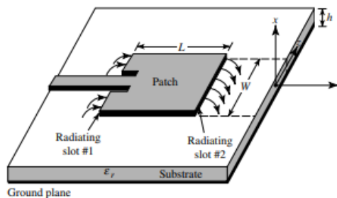
Gambar 1 Antena mikrostrip
