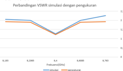
Gambar 10 Perbandingan nilai VSWR simulasi dengan pengukuran
