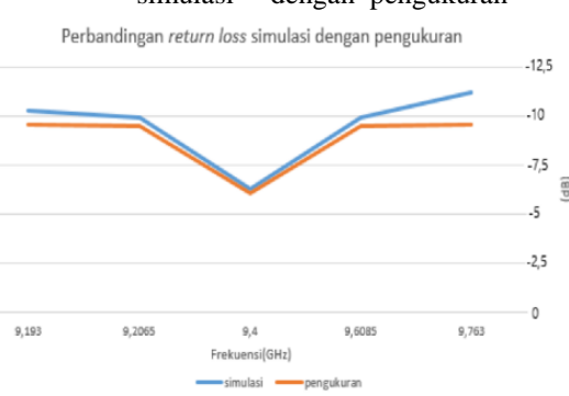
Gambar 12 Perbandingan nilai return loss simulasi dengan pengukuran
