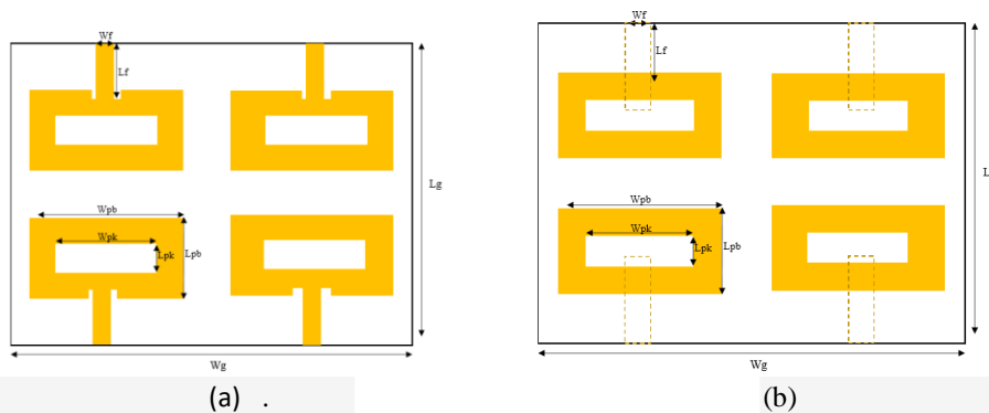
Gambar 3.1 Desain antenna MIMO 2x2 slot dual band pencatutan inset feed dan EMC
