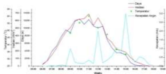
Gambar 4. 3 Grafik Rata-Rata Daya, Iradiasi, Temperatur Panel Surya, dan Kecepatan Angin Pada Rooftop
