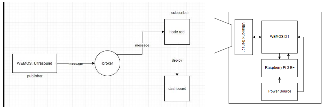
Gambar 1. Gambaran Umum Sistem dan gambaran alat
