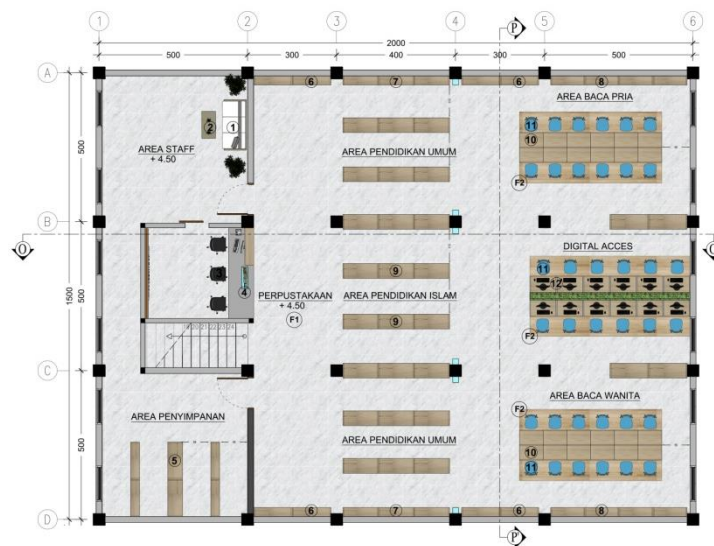
Gambar 7. Layout Perpustakaan
