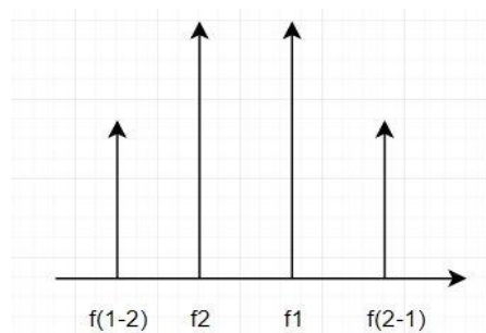
Gambar 2.1 Spektrum Frekuensi Akibat FWM
