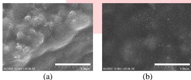
Gambar 3.9 Hasil uji SEM pada (a) rasio 1:1 dan (b) rasio 1:6 (serbuk:TETA)
