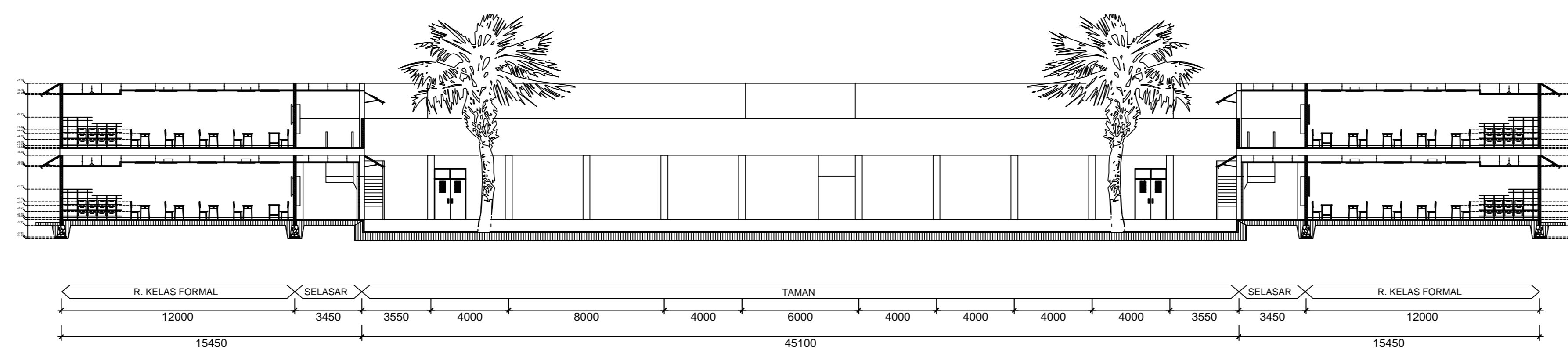
POTONGAN GENERAL B-B' SCALE: 1:100
