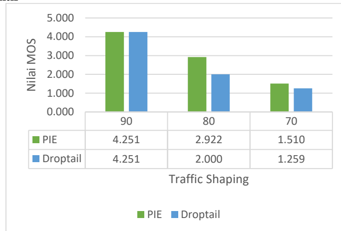
Gambar 7- MOS Objektif PIE dan Droptail
