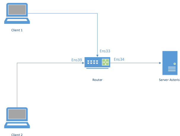
Gambar 2- Topologi
