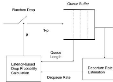
Gambar 1- Skema PIE
