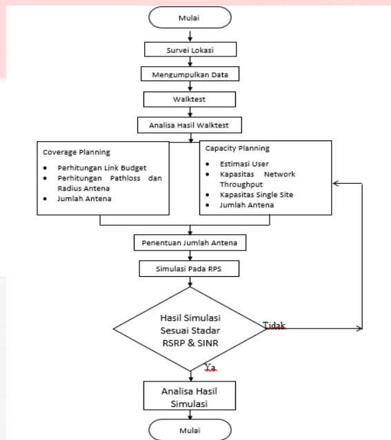
Gambar 3.1 Diagram Alir Perancangan Jaringan Femtocell
