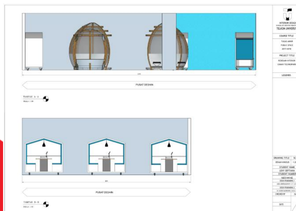
Gambar 16. Tampak Pusat Desain
