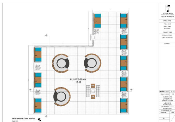
Gambar 15. Denah Khusus Pusat Desain
