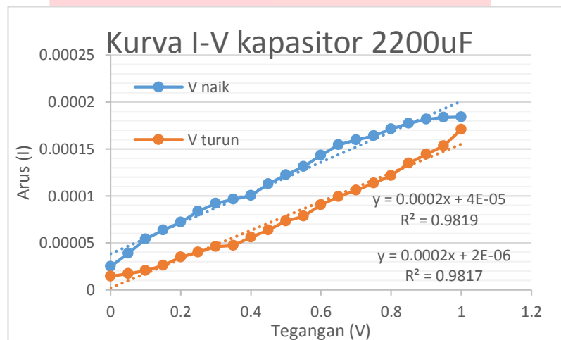
Gambar 4.2. Kurva Kapasitor 2200uF
