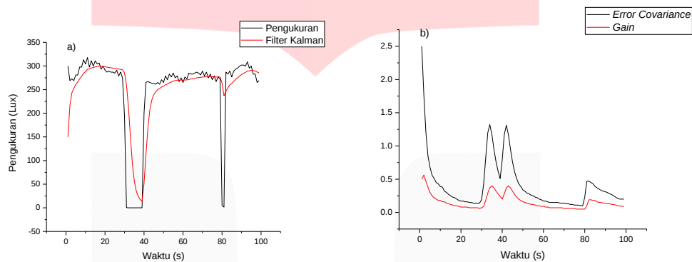
Gambar 4. 12 a) Grafik Respon Noise Cepat dan Lambat b) Grafik Gain Respon Noise Cepat dan Lambat
