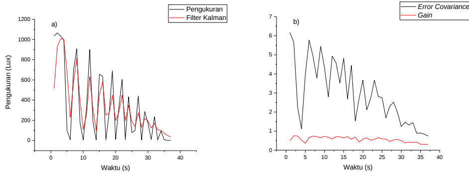
Gambar 4. 11 a) Grafik Penurunan Berulang Intensitas Cahaya per 10% b) Grafik Gain Penurun Berulang Intensitas Cahaya per 10%
