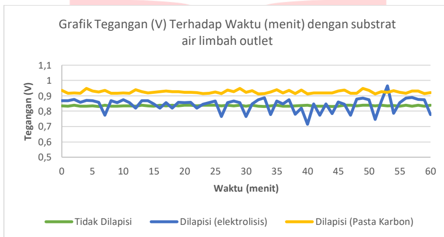
Gambar 3. 6 Grafik tegangan terhadap waktu dengan substrat air limbah outlet
