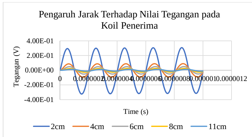
Gambar 4.4 Gelombang nilai tegangan penerima terhadap perubahan jarak.
