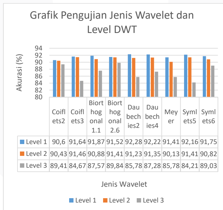
Gambar 5. Grafik Pengujian Jenis Wavelet Dan Level DWT
