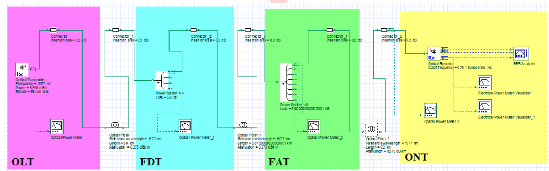
Gambar 3.9 Perancangan simulasi Link Downstream terjauh
