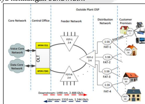
Gambar 2.4 Arsitektur XGPON [6]
