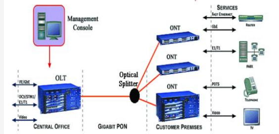
Gambar 2.3 Arsitektur FTTH [4]
