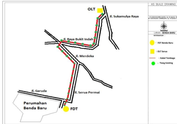
Gambar 3.2 Jalur Existing dari OLT sampai FDT
