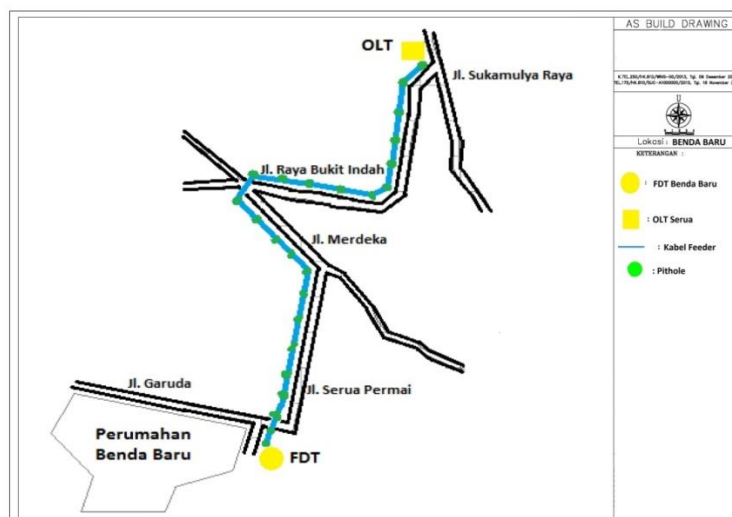
Gambar 3.5 Denah Perancangan dari OLT menuju FDT
