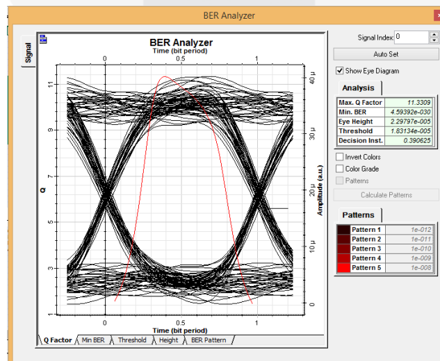
Gambar 4.1 Diagram mata Link Downstream terjauh
