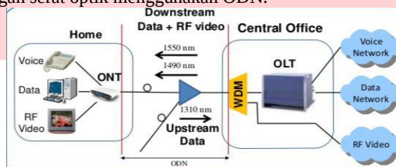
Gambar 2.2 Konfigurasi GPON [3]
