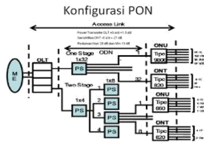
Gambar 2.1 Konfigurasi PON [3]
