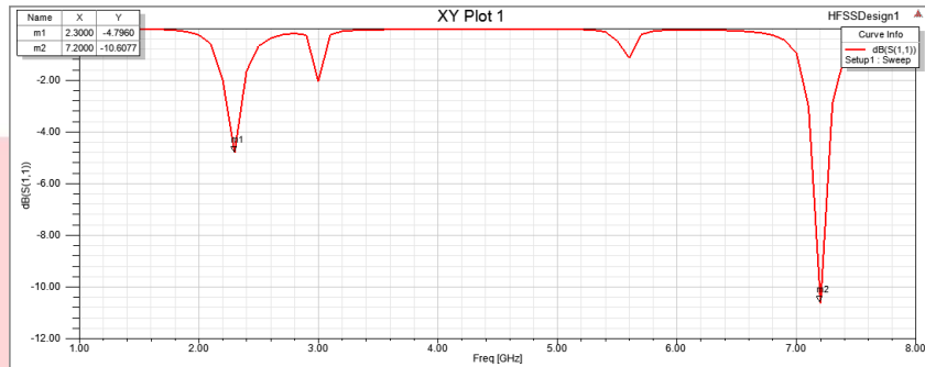
Gambar 3.3 Grafik S_{11} penyerap gelombang elektromagnetik berbasis AMC tanpa resistor
