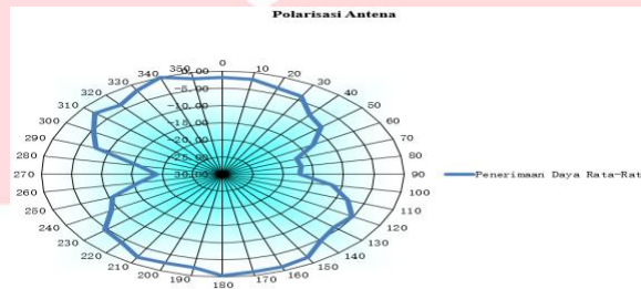
Gambar 9. Hasil pengukuran polarisasi antenna
