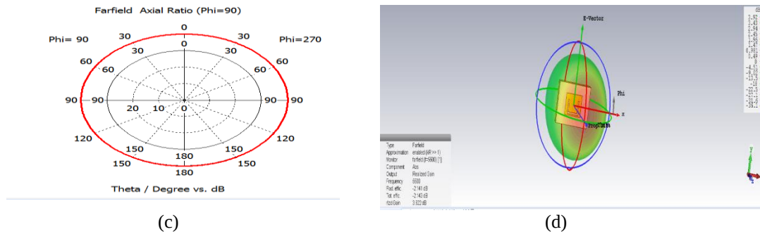
Gambar 6. Hasil Simulasi (a) pola radiasi azimuth (b) pola radiasi elevasi (c) polarisasi (d) gain
