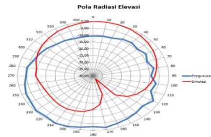
Gambar 8. Perbandingan hasil simulasi dan pengukuran pola radiasi elevasi
