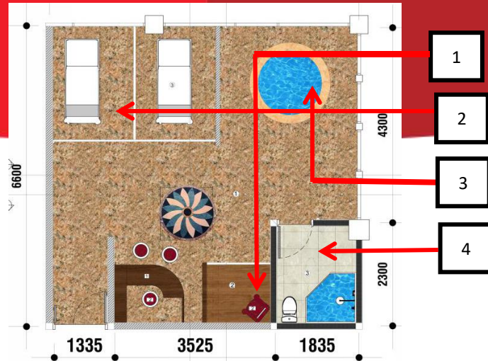
Gambar 12 : Alur Sirkulasi Aktivitas Ruang SPA VVIP
