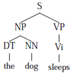
Gambar 1 Contoh Parser-tree
