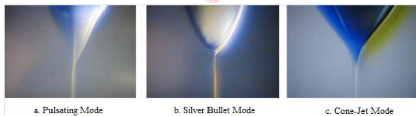
Gambar 2.1. Mode operasi sistem elektrospray
