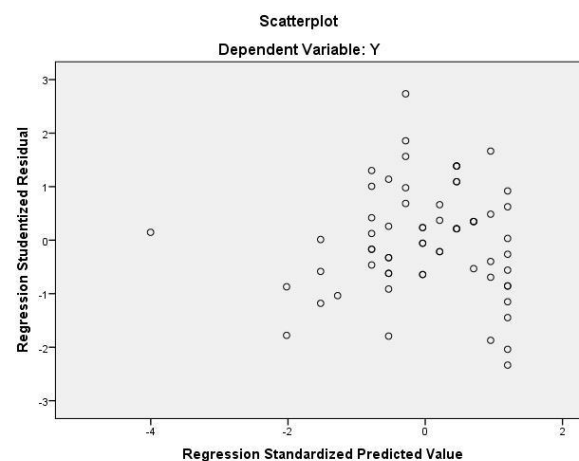
Gambar 3 Hasil Uji Heteroskedastisitas Sumber: Data Diolah, SPSS Versi 24
