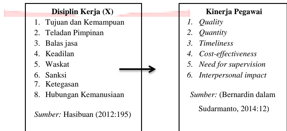
Gambar 1 Kerangka Pemikiran
